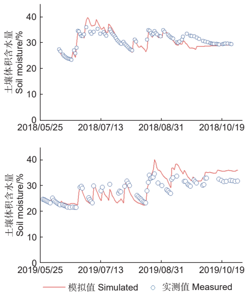
图 1 率定和检验期间华北落叶松人工林样地 0~60 cm 土层土壤体积含水量实测值与模拟值
