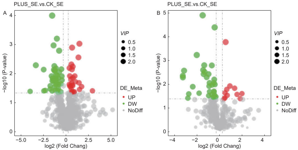
图 4 差异代谢物火山图。A-正离子化模式；B-负离子化模式
