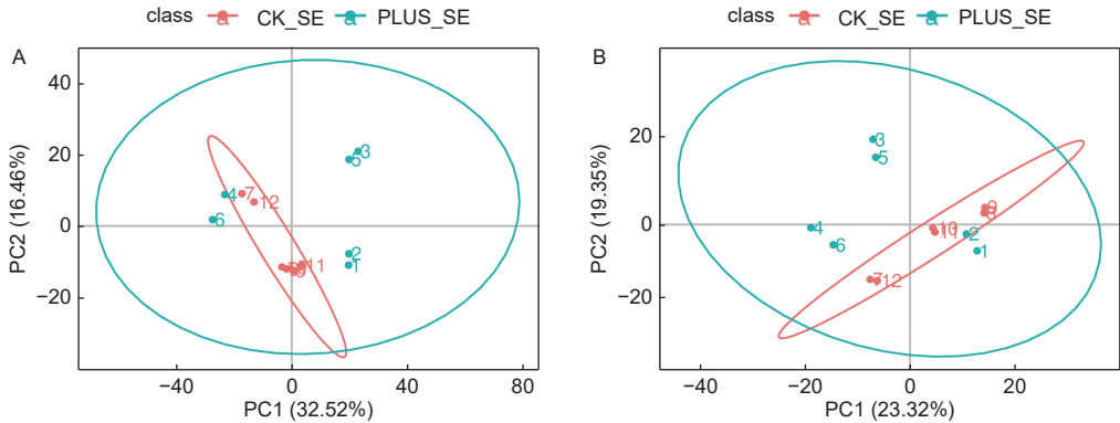
图 2 差异代谢物筛选的 PCA 分析。A-正离子模式；B-负离子模式。CK_SE 为对照，PLUS_SE 为硒处理。QC 为质控
