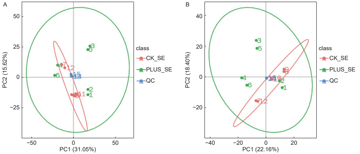
图 1 总样本 PCA 分析。A-正离子模式；B-负离子模式。CK_SE 为对照，PLUS_SE 为硒处理。QC 为质控
